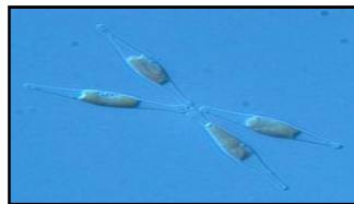
Phaeodactylum
