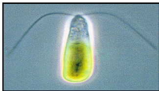
Dunaliella
