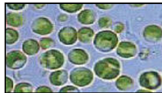
Nannochloropsis
