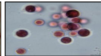
Porphyridium
