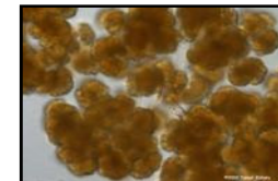
Botryococcus
