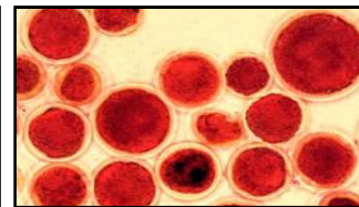
Haemotococcus
